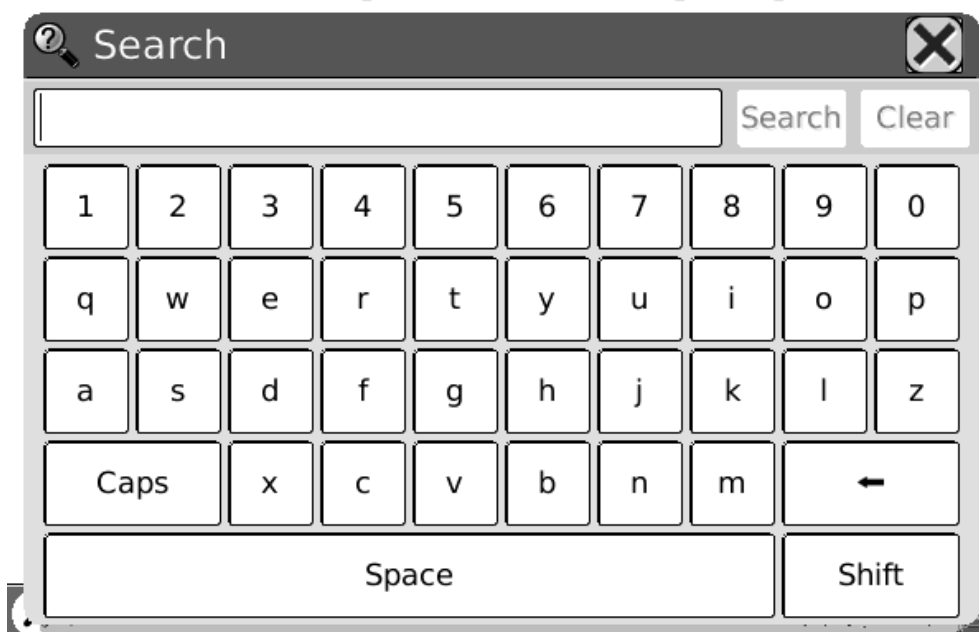
Fig. 7.4.12.1 (1) Invoeren zoekopdracht
