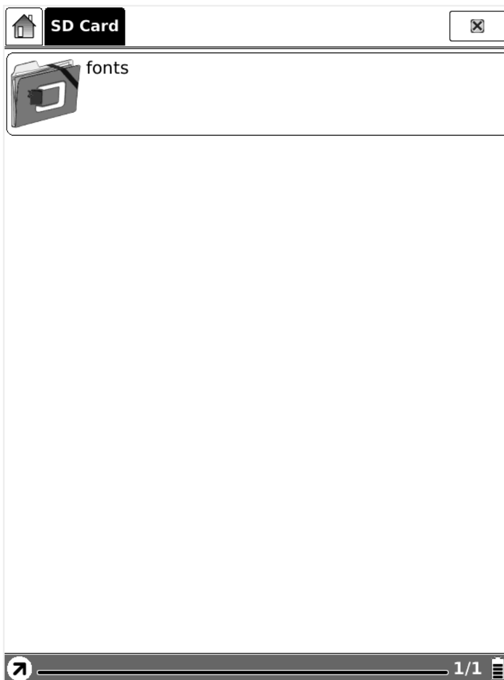
Fig. 7.4.6.2 (2) Zoekresultaten
