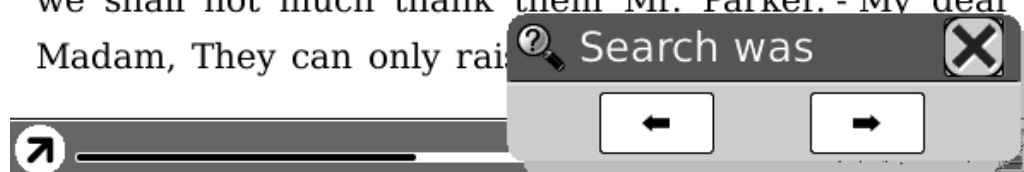
Fig. 7.7.1.2 (1) Tekst zoekresultaat
