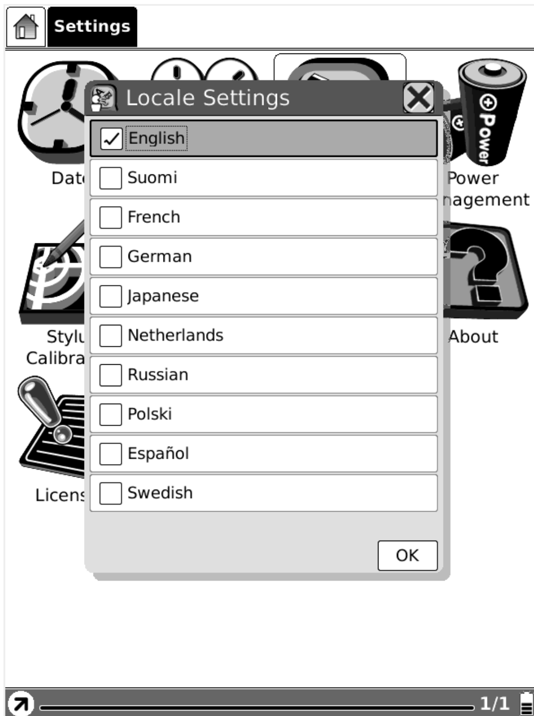
Fig. 7.1.6.3 Lokaal dialoogvenster
