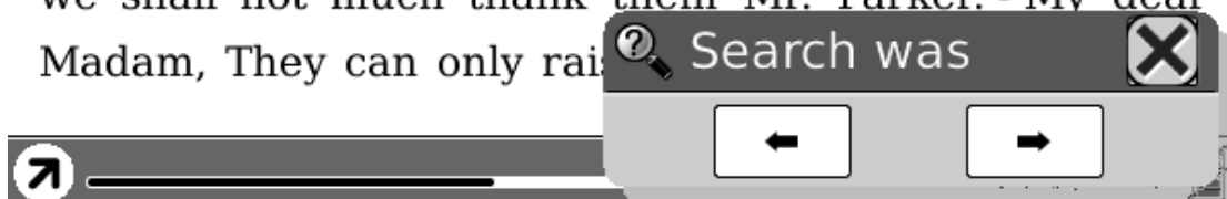
Fig. 7.4.12.1 (2) Tonen zoekresultaten
