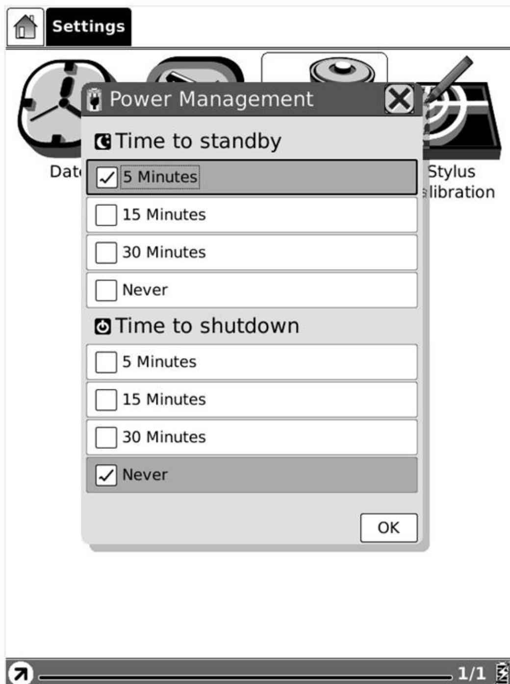
Fig. 7.1.6.4 Energiebeheer
