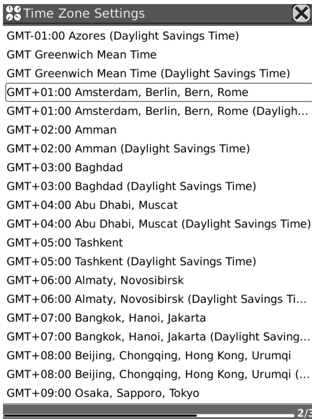
Fig. 7.1.6.2 Tijdzone instellingen
